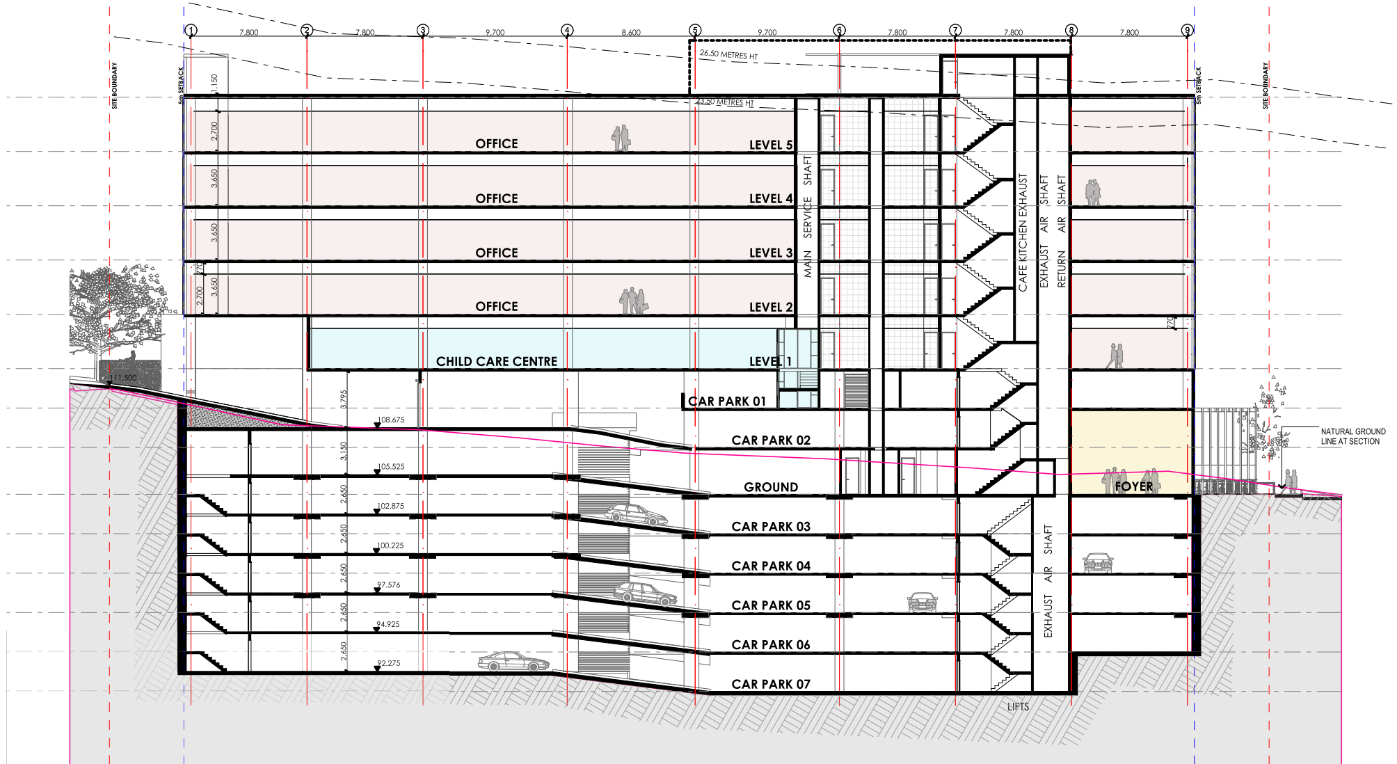
A SECTION A 11013 DA 01a.rvt SCALE 1:250
